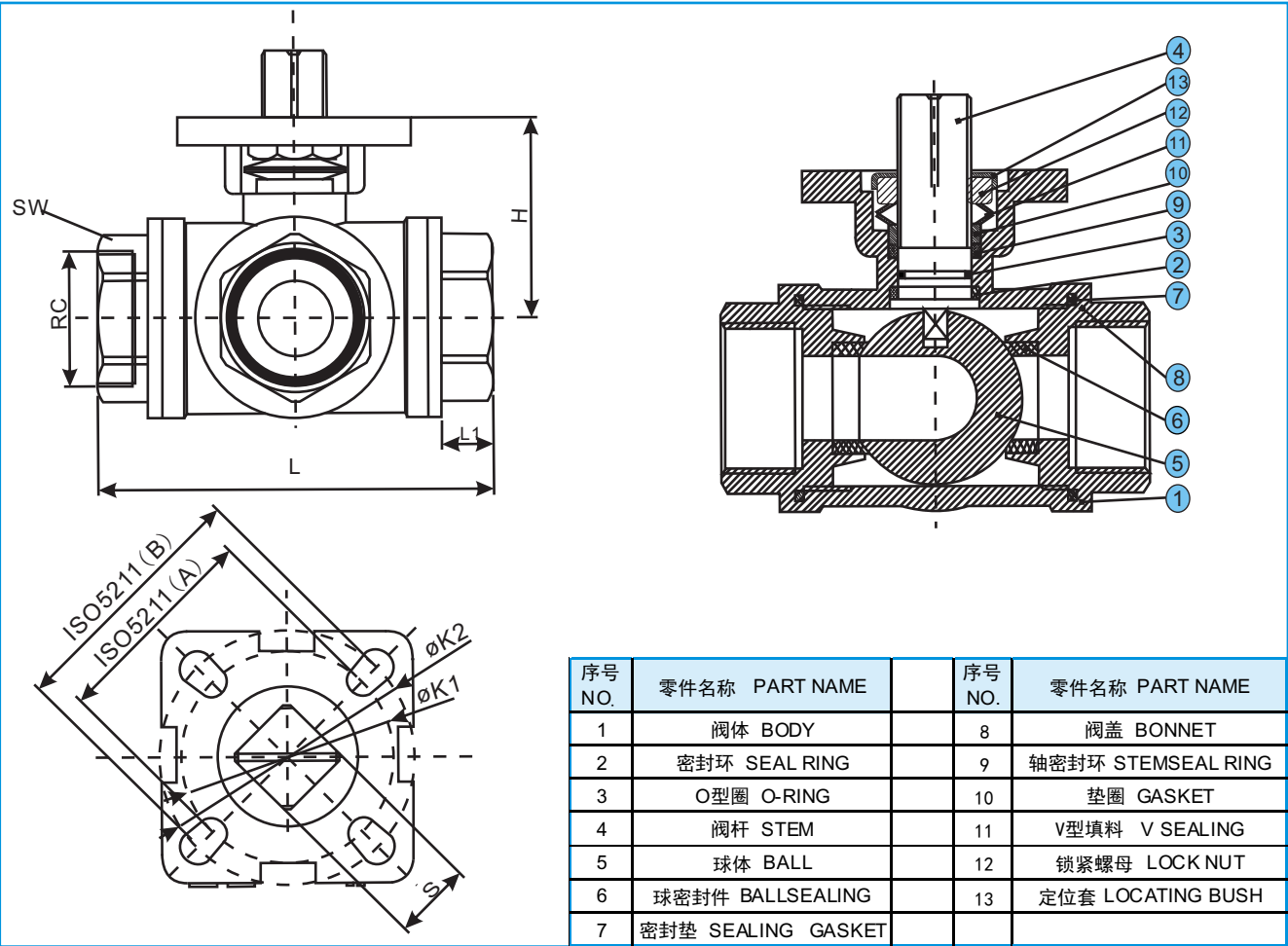
外形尺寸(单位:mm)
